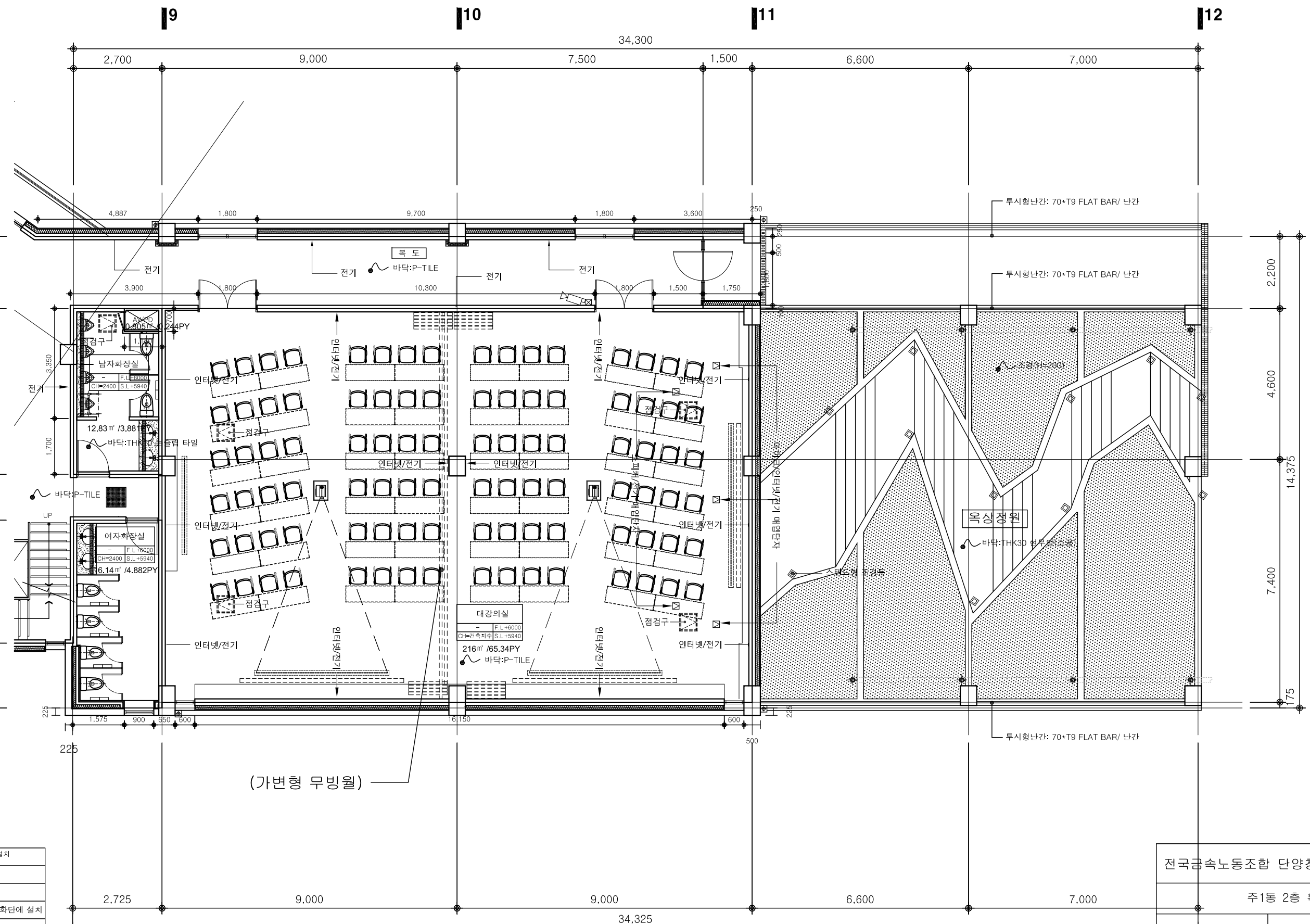
주1동 2층 확대 평면도-2
